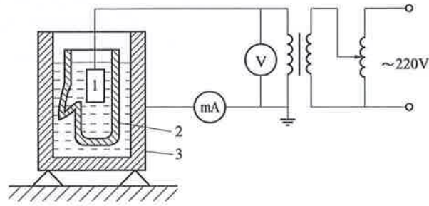
图 B.4 辅助型绝缘手套试验接线图
